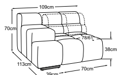
Element 70 s područkou AT-L s nastavitelnou hloubkou sedu RVM Typ. číslo: D021104
