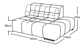
Ukončovací díl P s nastavitelnou hloubkou sedu RVM Typ. číslo: D021521
