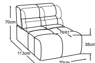
Element 70 s nastavitelnou hloubkou sedu RVM Typ. číslo: D021118
