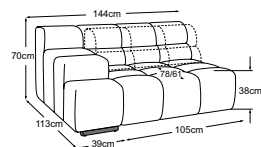
Element 105 s područkou AT-L s nastavitelnou hloubkou sedu RVM Typ. číslo: D021106
