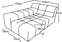
Prodloužená pohovka L s prodlouženou područkou Typ. číslo: D021119
