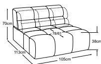
Element 105 s nastavitelnou hloubkou sedu RVM Typ. číslo: D021117
