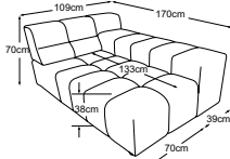
Prodloužená pohovka P s prodlouženou područkou Typ. číslo: D021120
